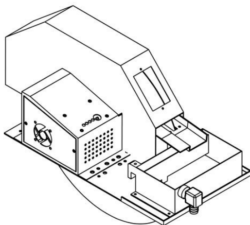
DG-400 TSL. 外觀尺寸表
